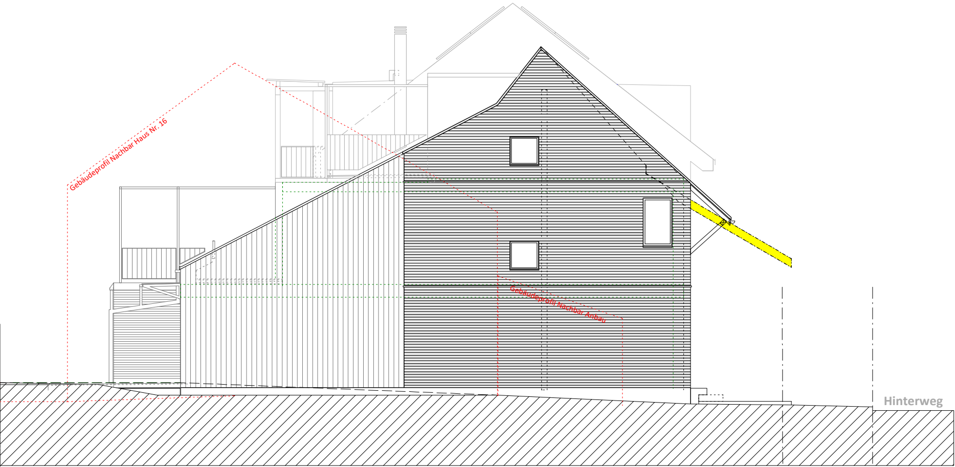
Fassade Nord-Ost (Grenze zu Nachbar)
